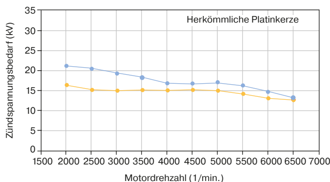
Zündspannungsbedarf steigt im Gasbetrieb
